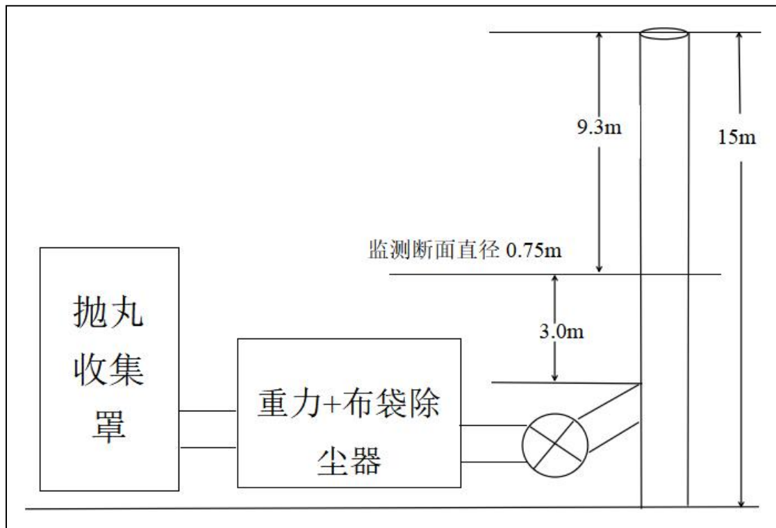
(13) DA045 5线抛丸排气筒监测点位示意图
