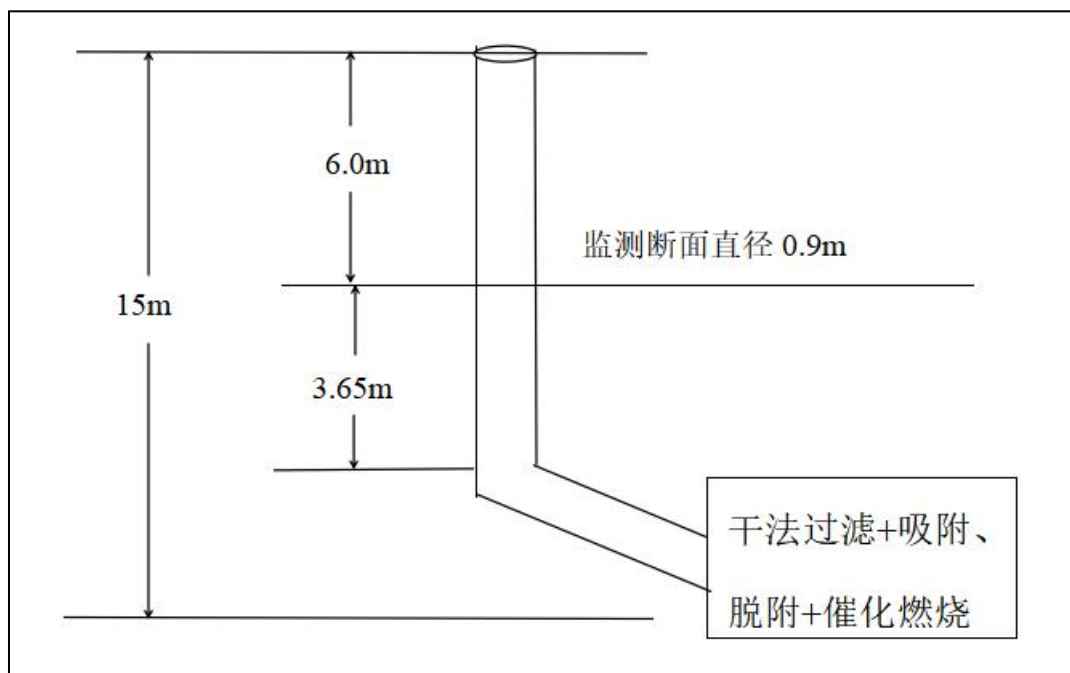
(18) DA009 5线喷涂、烘干监测点位示意图
