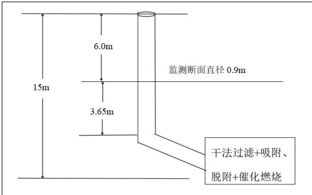
(15) DA014 2线喷涂、烘干监测点位示意图
