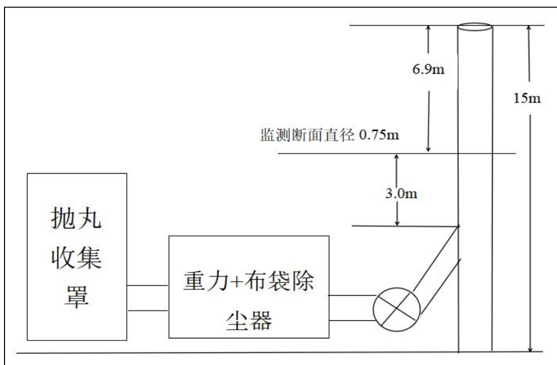
(9) DA042 1线抛丸排气筒监测点位示意图
