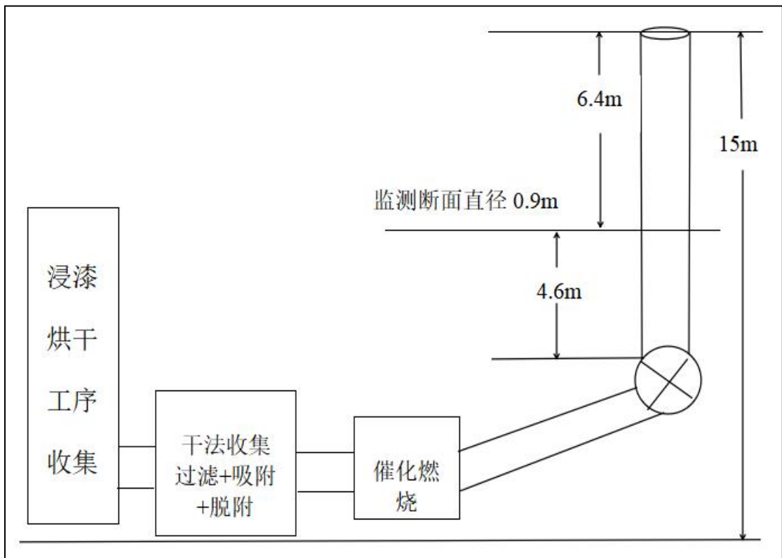
(31) DA028 管件涂装浸漆线 (1#) 监测点位示意图
