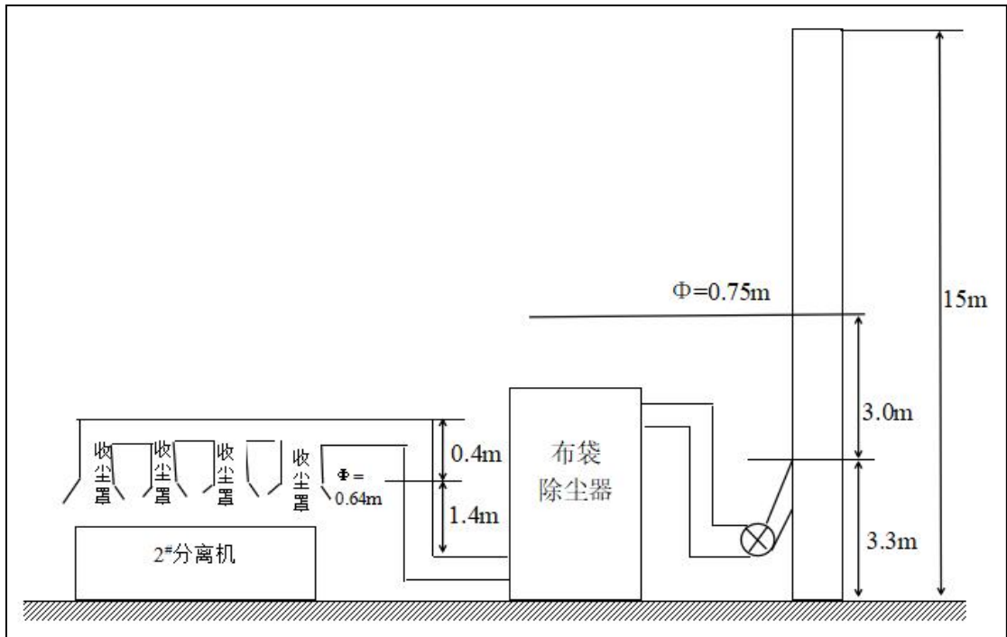
(29) DA039 2#分离工段监测点位示意图
