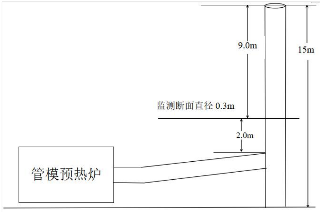
(20) DA066 管模预热炉烟气监测点位示意图
