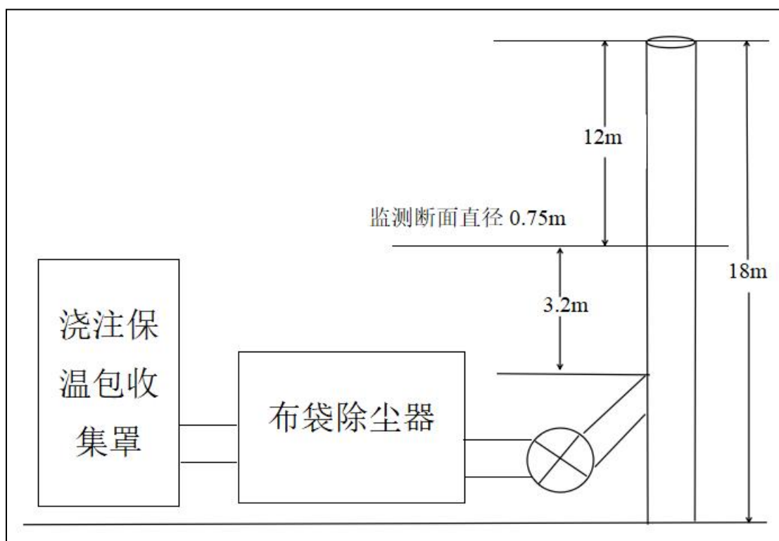
(8) DA046 浇铸保温包排气筒监测点位示意图
