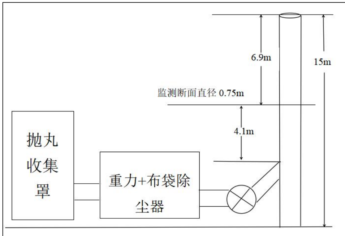
(10) DA031 2线抛丸排气筒监测点位示意图
