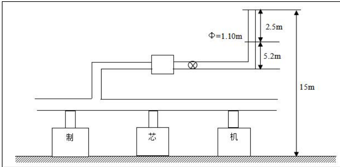
(24) DA061 27#-34#制芯机监测点位示意图
