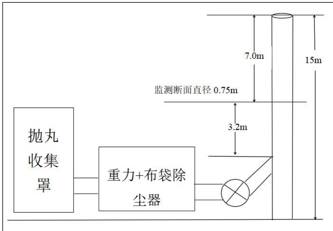
(11) DA035 3线抛丸排气筒监测点位示意图
