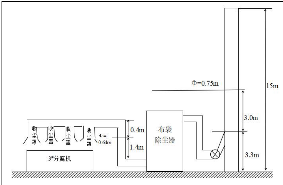
(30) DA043 3#分离工段监测点位示意图
