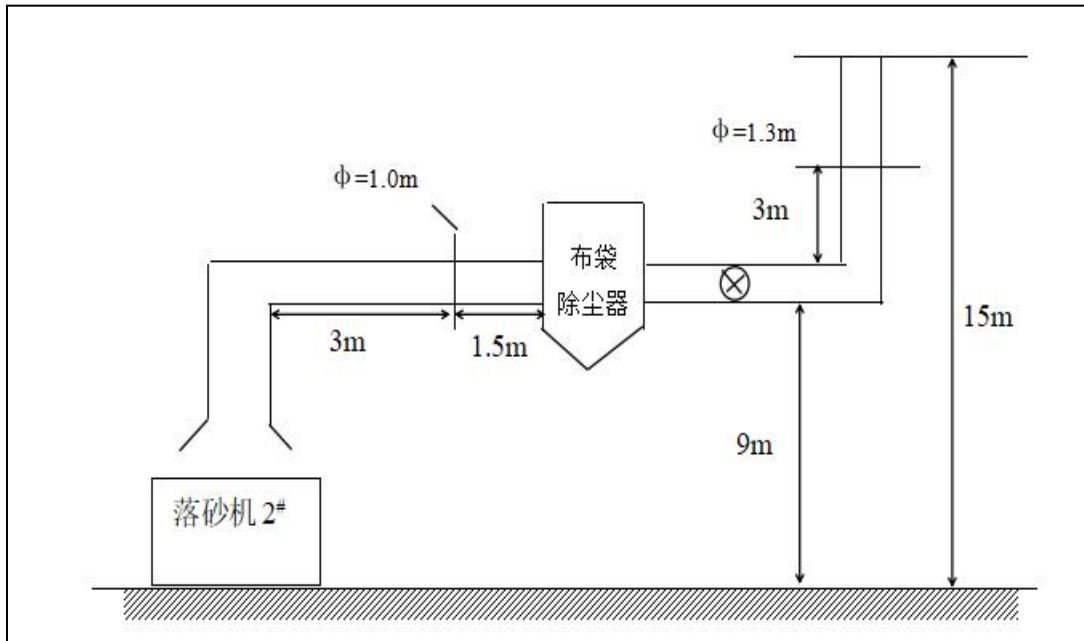
(26) DA020 造型、落砂 2#监测点位示意图
