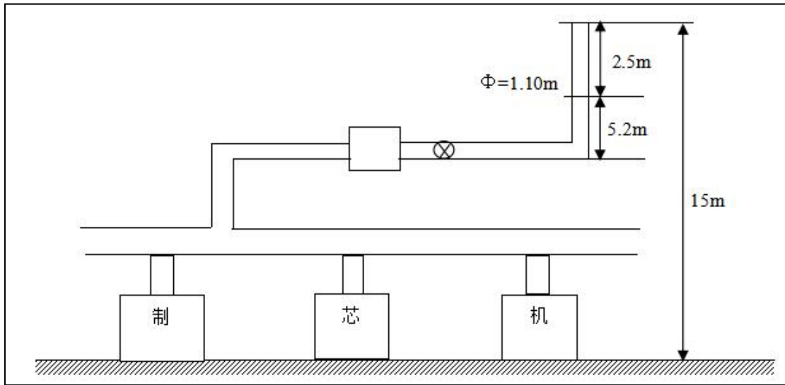
(22) DA059 1#-12#制芯机监测点位示意图
