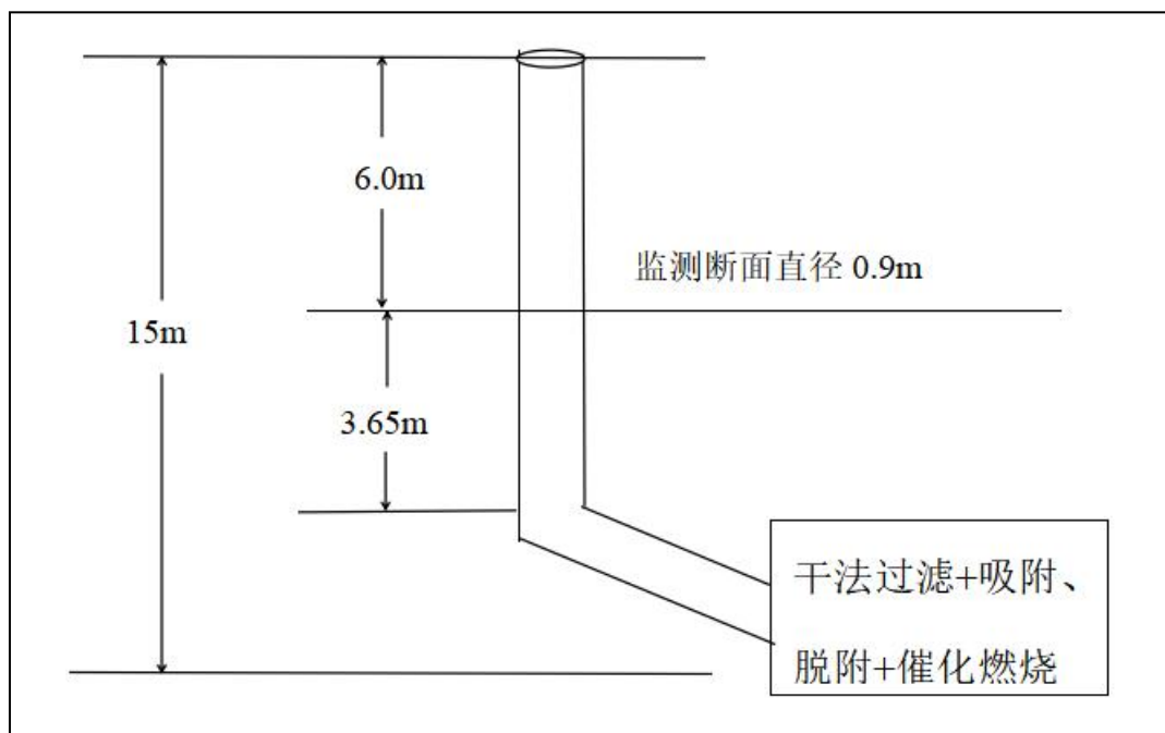
(16) DA005 3线喷涂、烘干监测点位示意图
