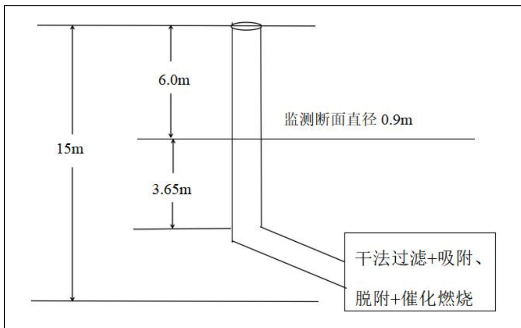
(17) DA018 4线喷涂、烘干监测点位示意图
