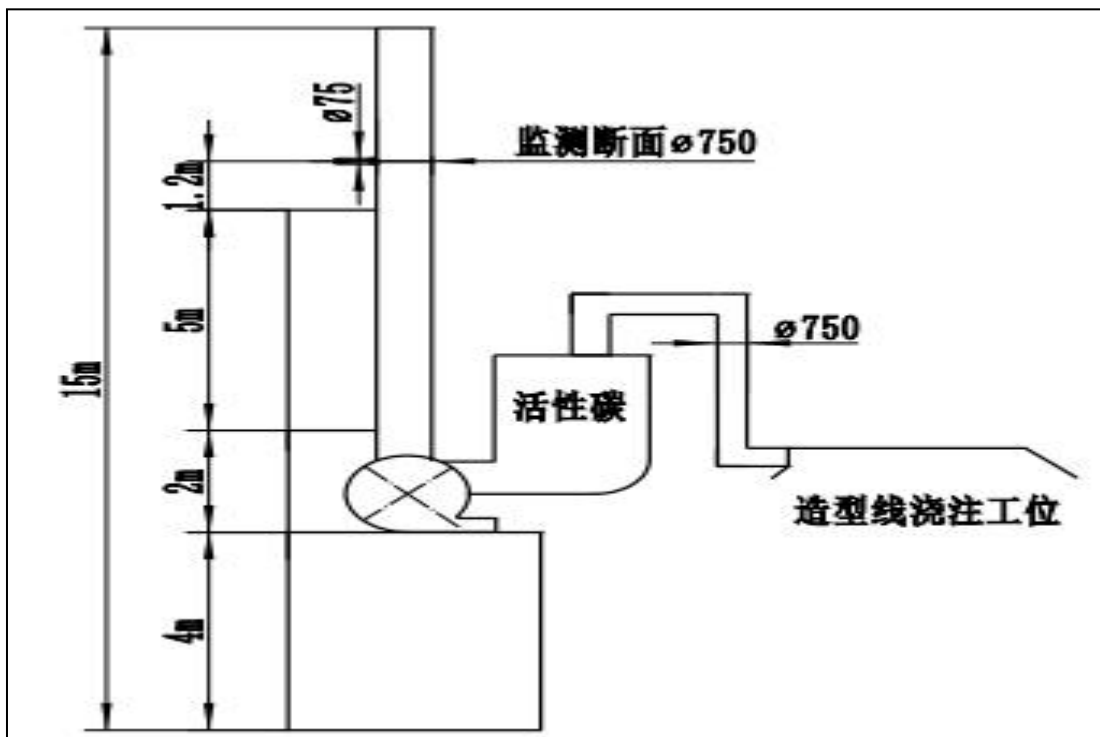
(33) DA011 浇铸工位 1#监测点位示意图
