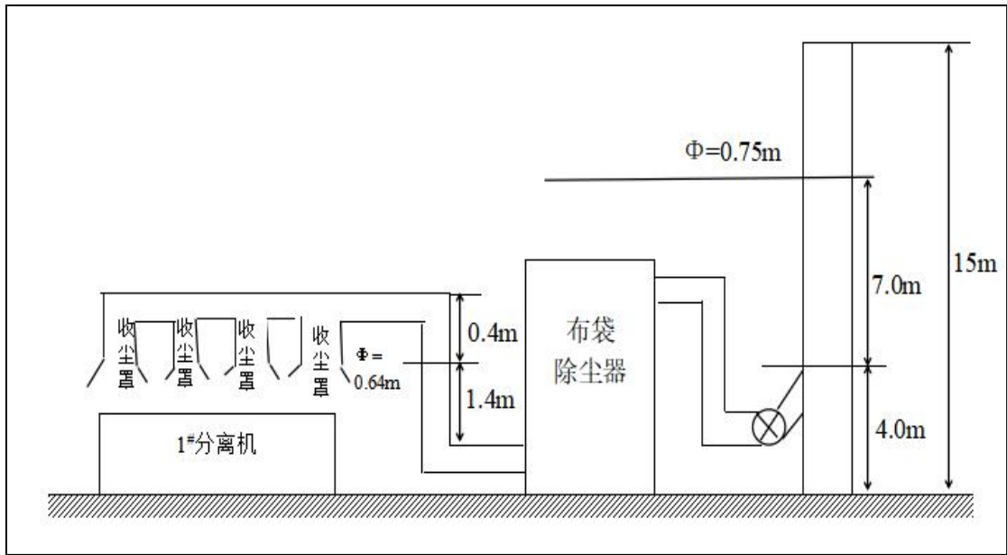
(28) DA044 1#分离工段监测点位示意图
