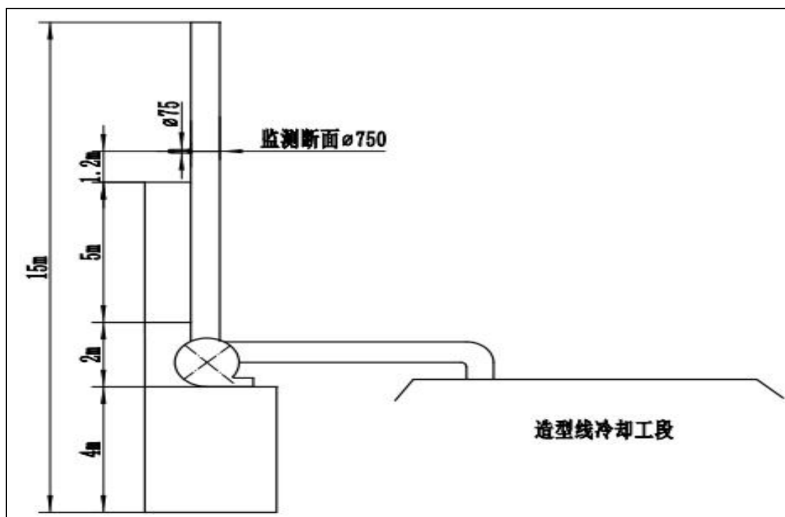
(38) DA012 造型冷却工位 1#监测点位示意图
