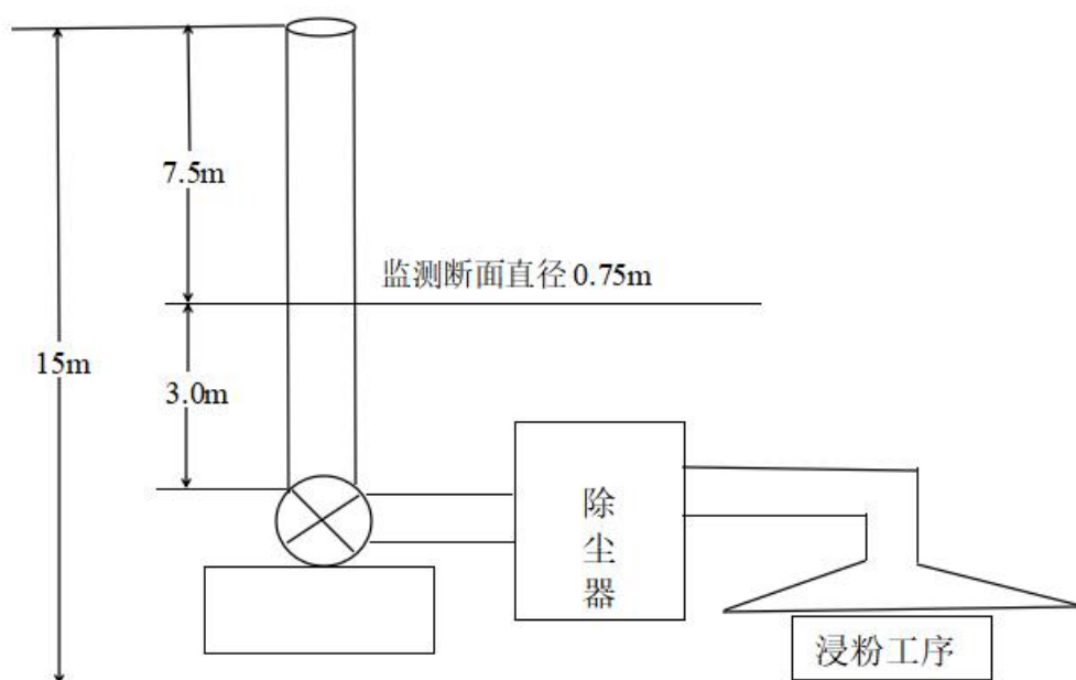
(43) DA030 管件涂装浸漆线 (1#) 浸粉监测点位示意图
