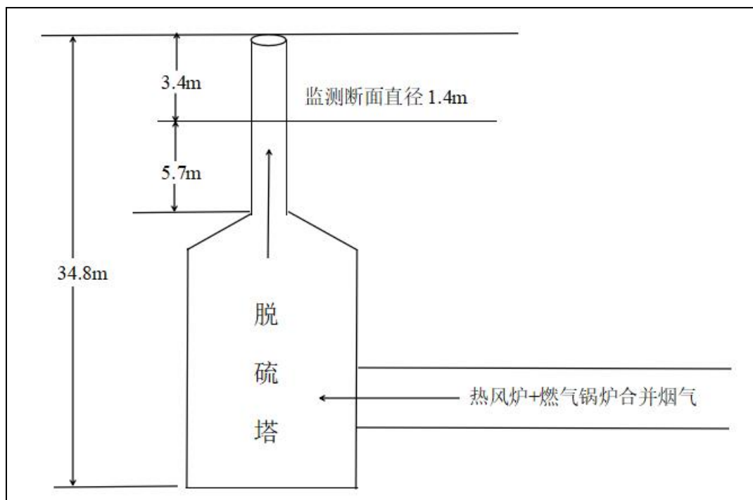
(2) DA055 高炉热风炉烟气监测点位示意图
