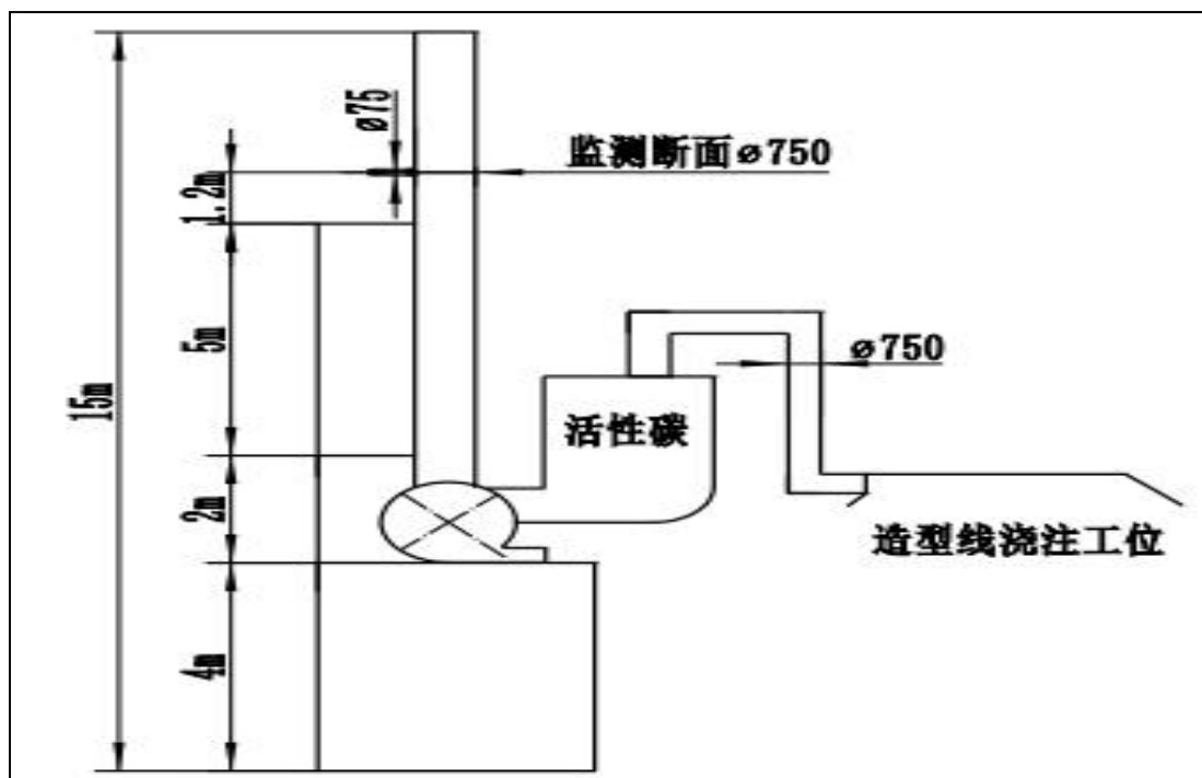
(36) DA007 浇铸工位 4#监测点位示意图
