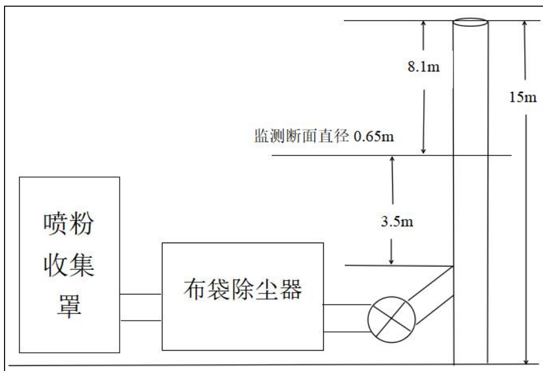
(19) DA027 2#喷粉线监测点位示意图
