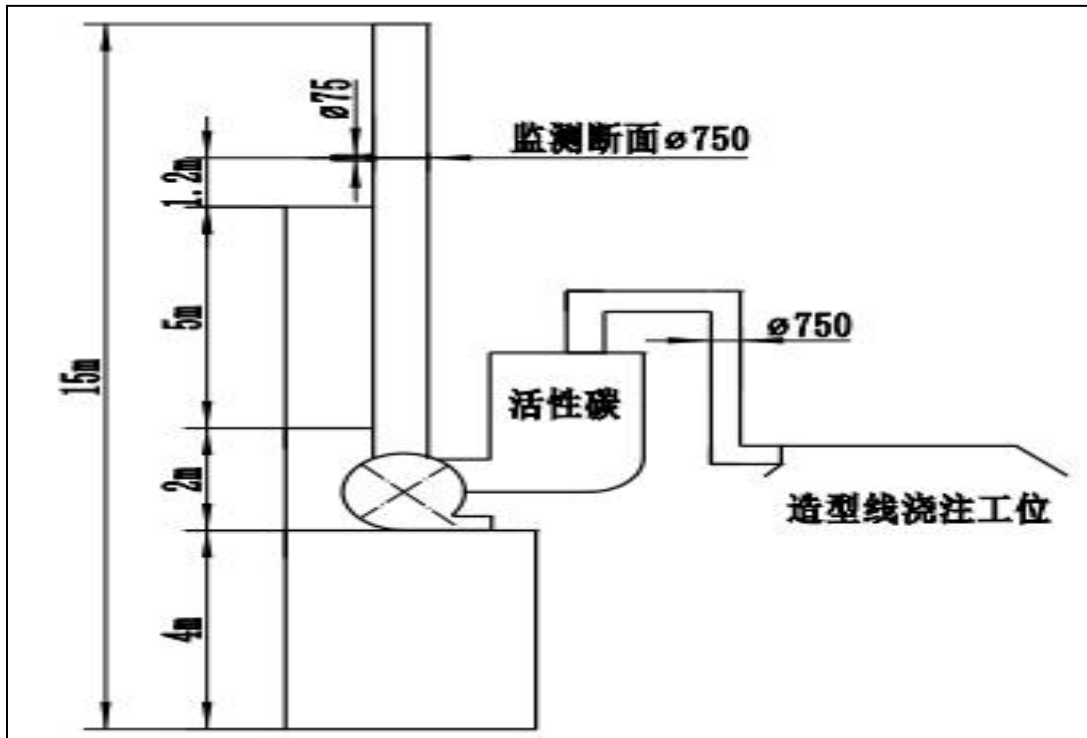
(34) DA021 浇铸工位 2#监测点位示意图
