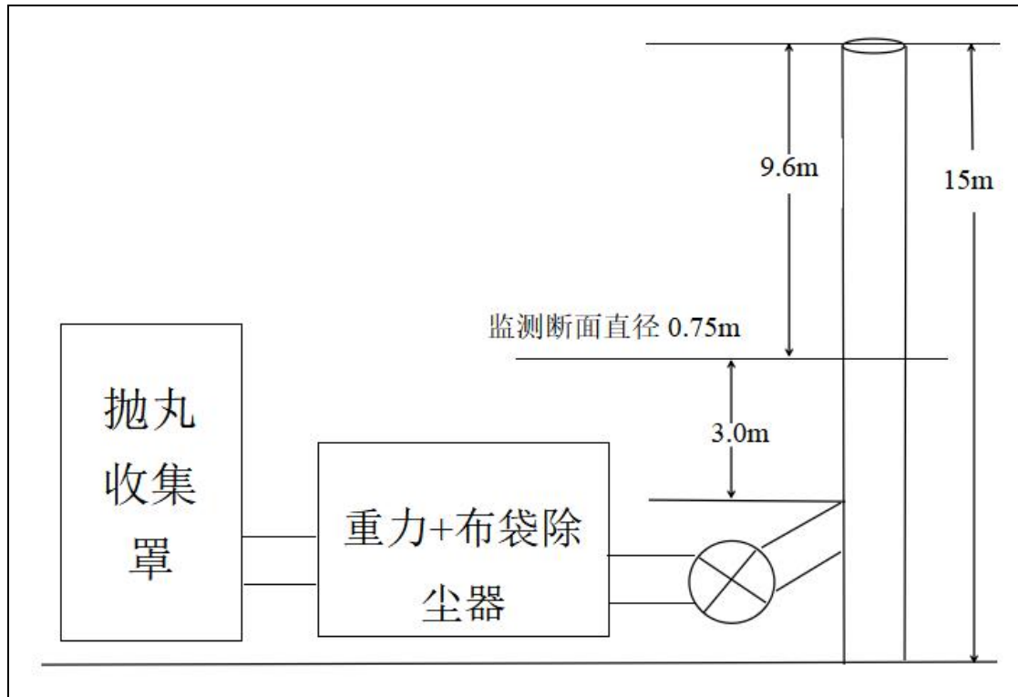
(12) DA029 4线抛丸排气筒监测点位示意图
