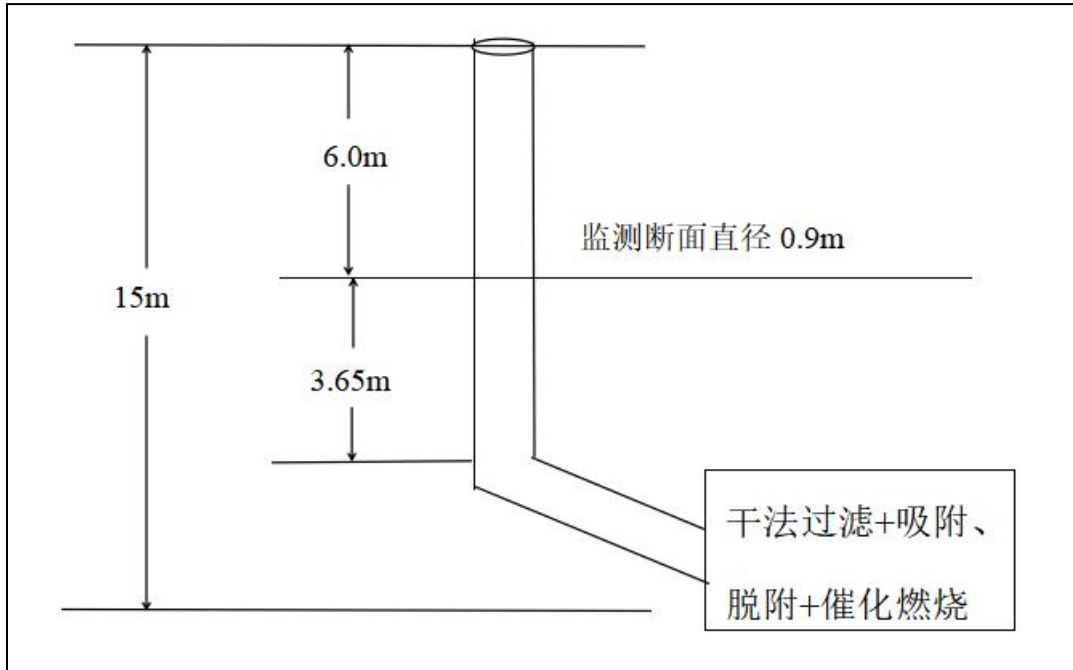
(14) DA023 1线喷涂、烘干监测点位示意图
